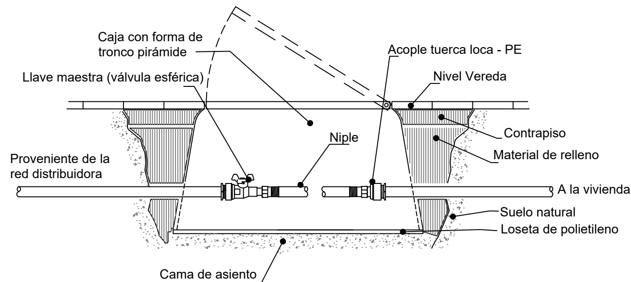
DESPIECE CONEXIÓN DOMICILIARIA
