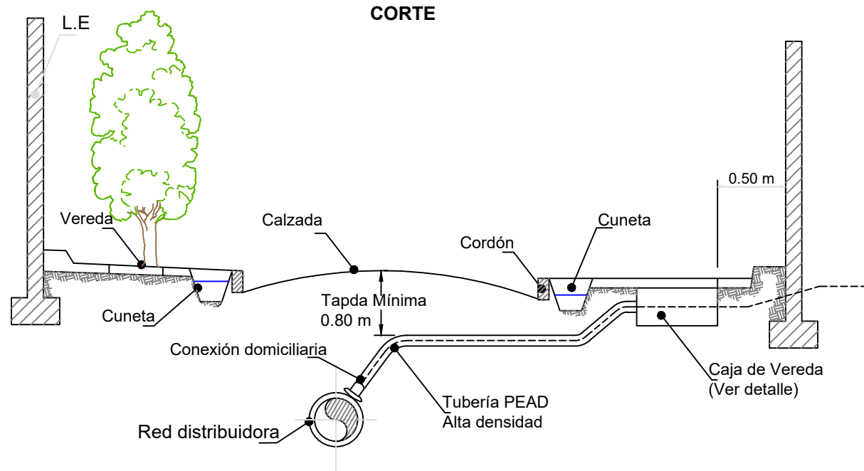
ESQUEMA CAJA PARA CONEXIÓN DOMICILIARIA Y LLAVE MAESTRA
