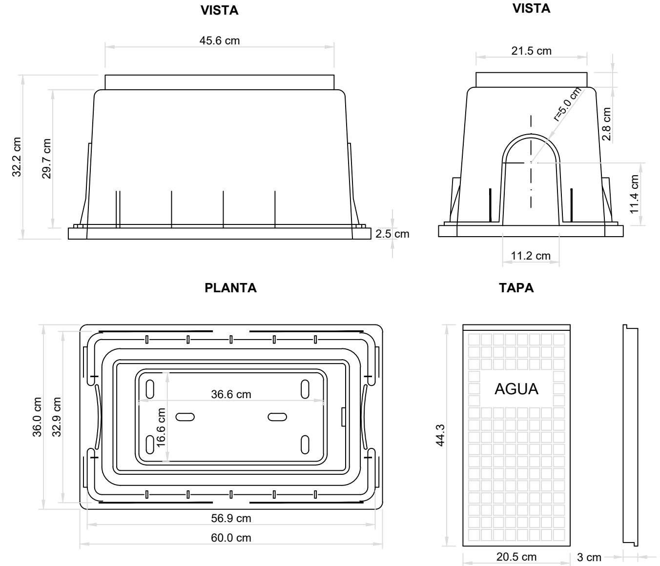
DETALLE DE CAJA PARA VEREDA
